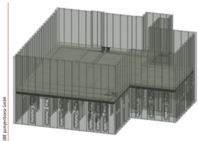
Abb. 5 - Thermisch aktivierte Schlitzwand mit BIM
